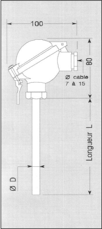
Thermocouple Classe II, L = selon type, tête Standard aluminium type TS
